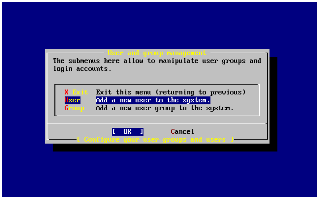
图 51. 选择用户
